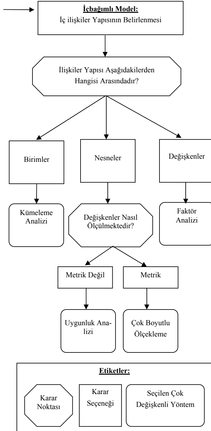
Şekil 2.1: Çok Değişkenli Bir Yöntemin Seçimi (Devam)
