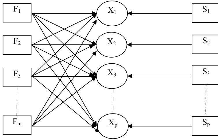
Şekil 2.13: Çok Faktörlü Yapıların Şematik Gösterimi
