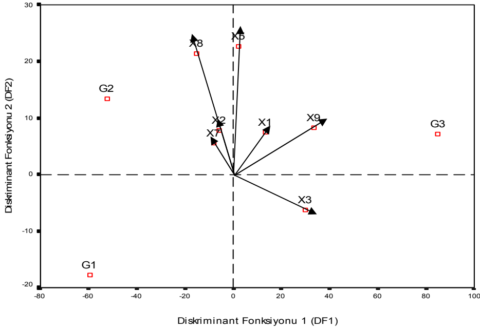
Şekil 2.33: İndirgenmiş Diskriminant Uzayında Genişletilmiş Özellik Vektörleri 254
