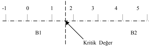
Şekil 2.26: Diskriminant Değerlerinin Tek Boyutlu Grafiği
