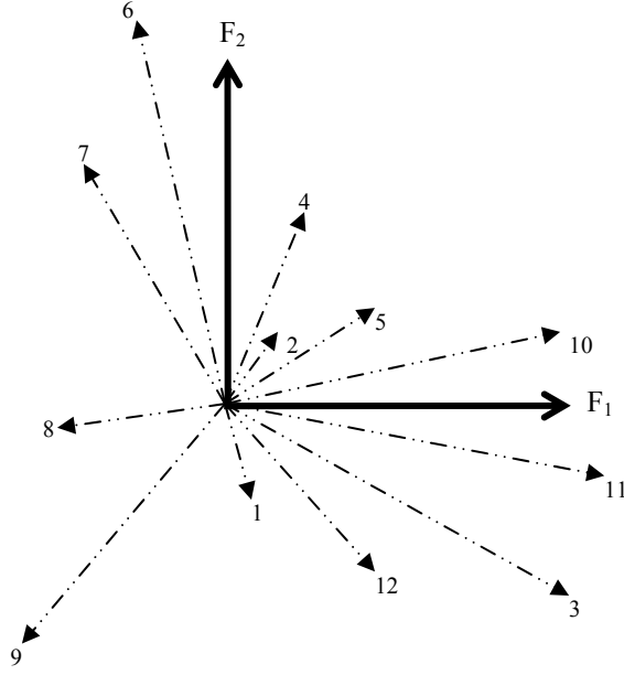
Şekil 2.14: İki Faktörlü ve 12 Değişkenli Bir Modelin Geometrik Gösterimi
