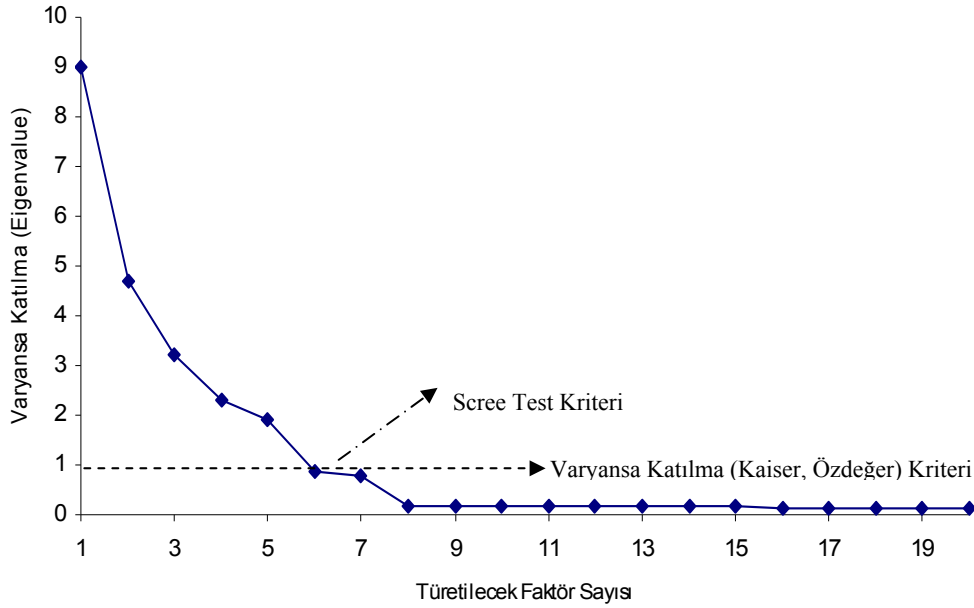
Şekil 2.8: Scree Testi ve Varyansa Katılma (Kaiser) Kriteri
