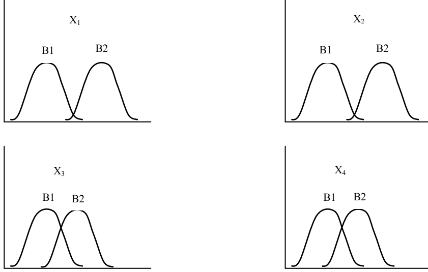
Şekil 2.24: Teorik Değişkenlerin Dağılımı 181
