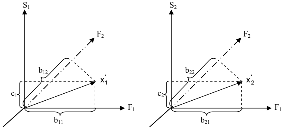
Şekil 2.19: Ortak Varyans Tahmini ve Faktör Belirsizliği 155
