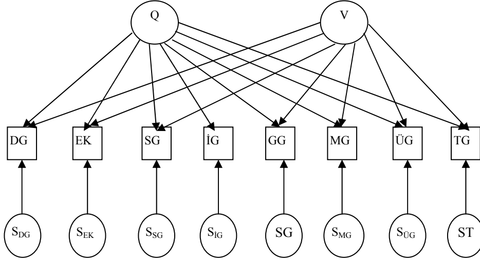
Şekil 2.6: Gelişmişlik ile Göstergeler Arasındaki İlişki (İki-Faktörlü Model)
