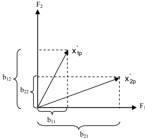
Şekil 2.20: İki Boyutlu Alt Faktör Uzayında Vektörlerin İzdüşümü
