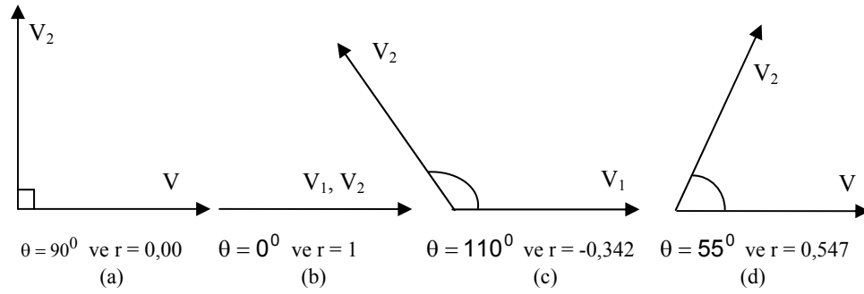
Şekil 2.11: Korelasyon Katsayılarının Açılı ve Vektörlerle Gösterilmesi
