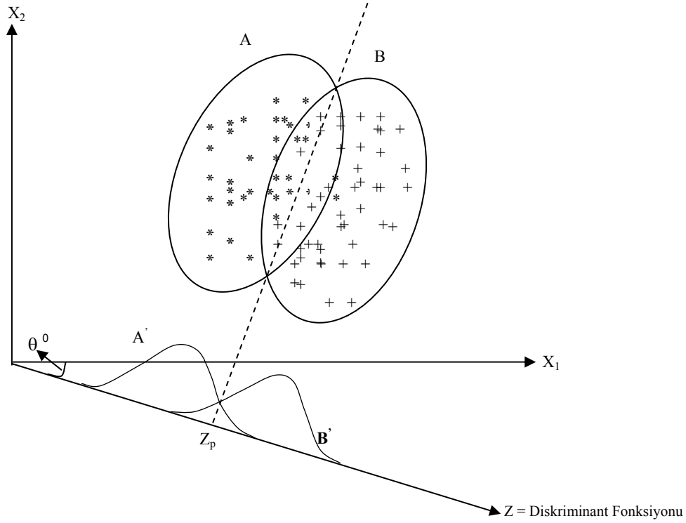
Şekil 2.22: İki Grulu Diskriminant Analizinin Grafik Gösterimi
