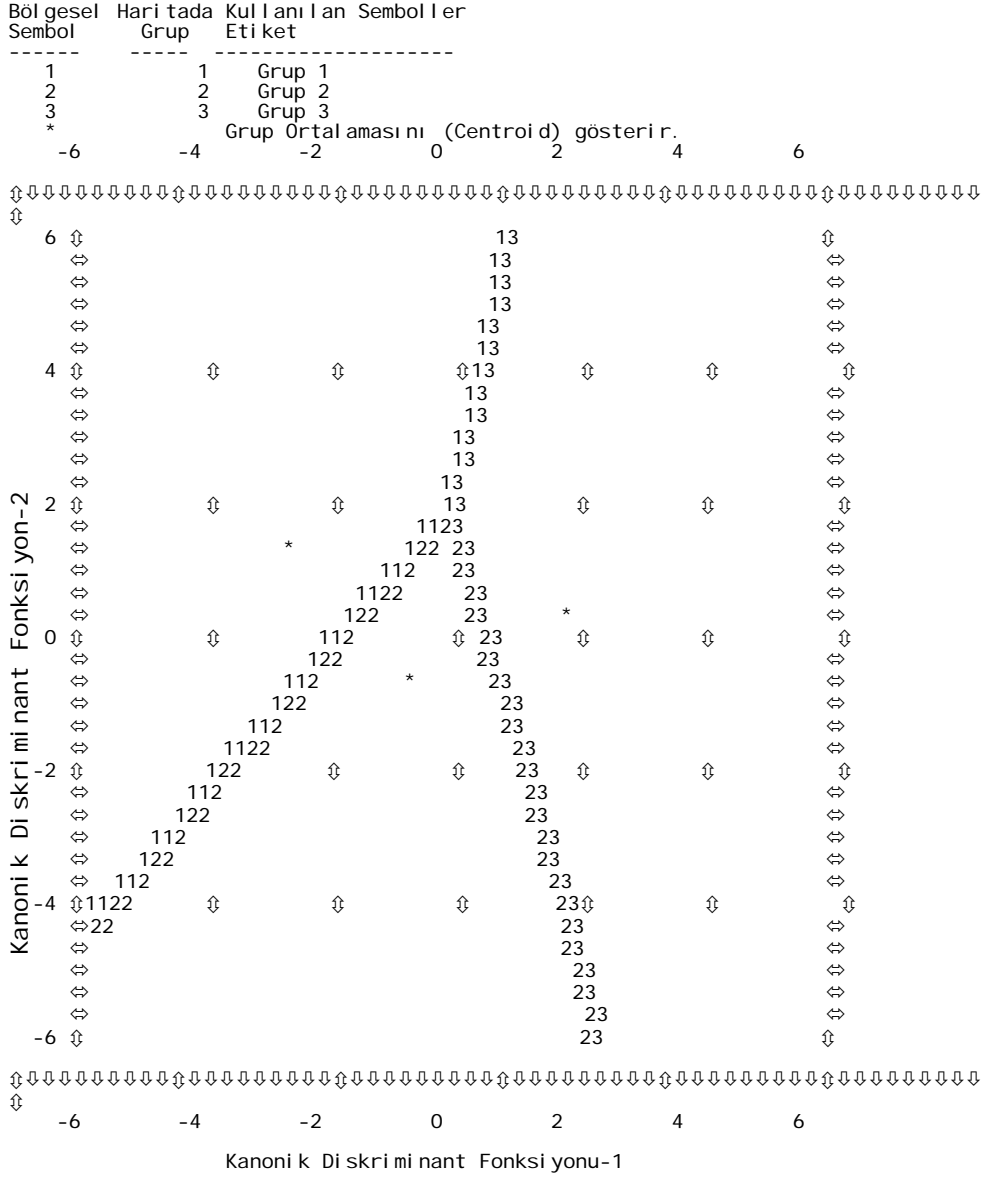
Şekil 2.34: Bölgesel Harita (Territorial Map)
