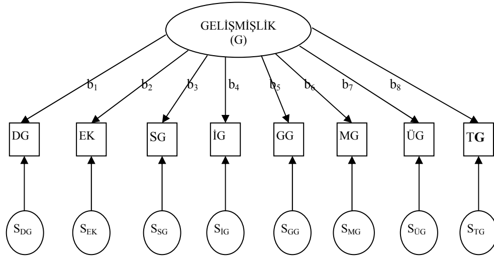
Şekil 2.5: Gelişmişlik ile Göstergeler Arasındaki İlişki (Tek-Faktörlü Model)
