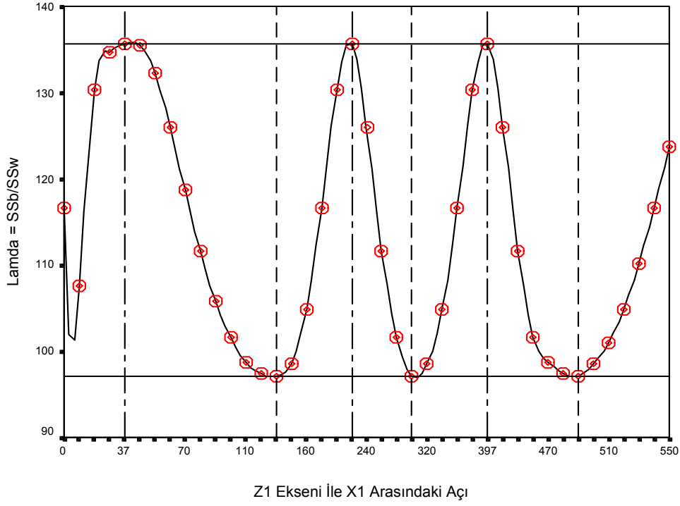
Şekil 2.30: Lamda Değerleri ile Değişik Rotasyon Açılı Grafiği
