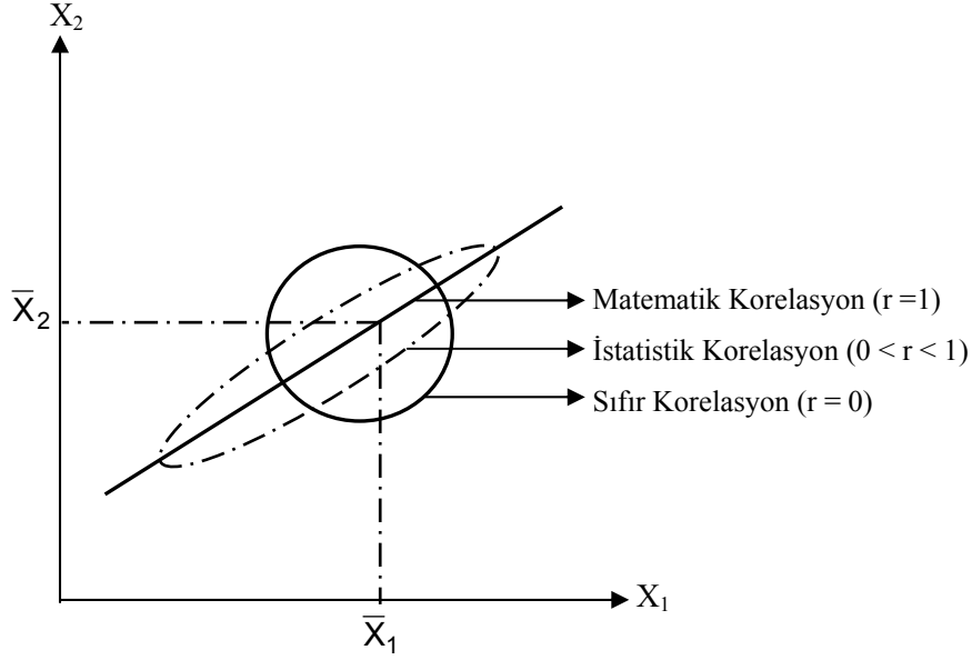
Şekil 2.10: Korelasyon Katsayısının Geometrik Gösterimi
