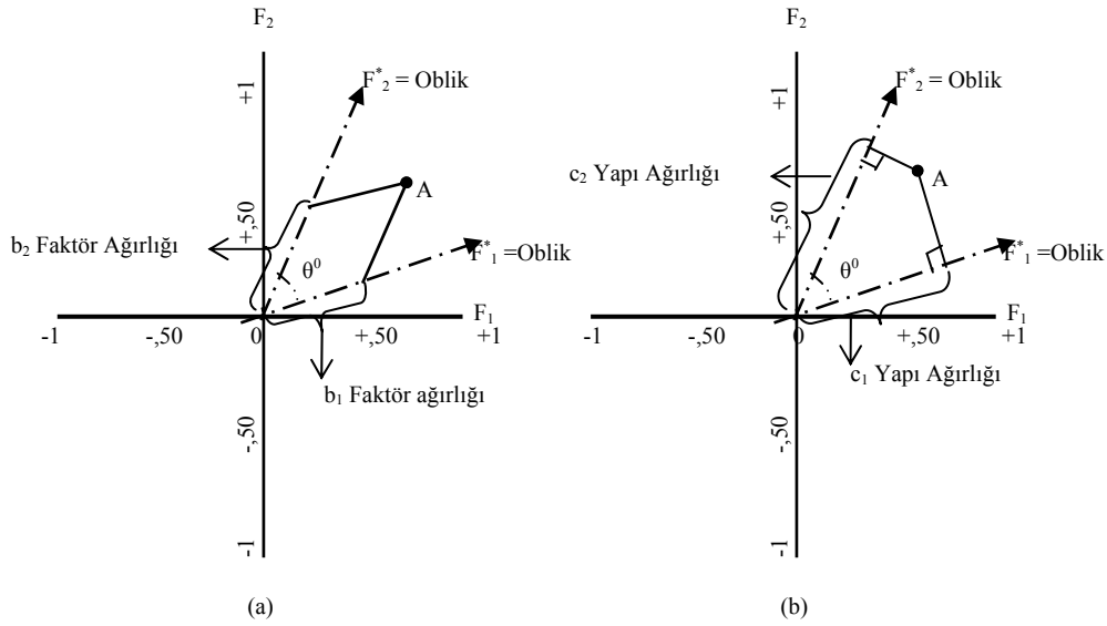
Şekil 2.16: Oblik (Eğik, Bağımlı) Faktör Rotasyonu: Faktör ve Yapı Ağırlıkları
